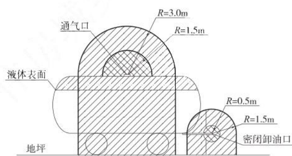
图 C.0.4 汽油油罐车的爆炸危险区域划分 0区； 1区； 2区
