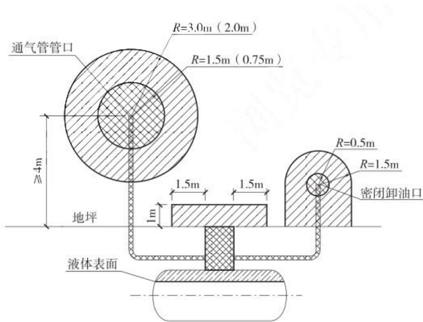
图 C.0.3 汽油埋地卧式油罐的爆炸危险区域划分
